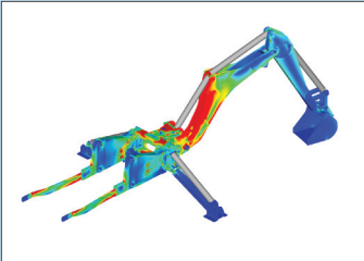
Linear Statics
